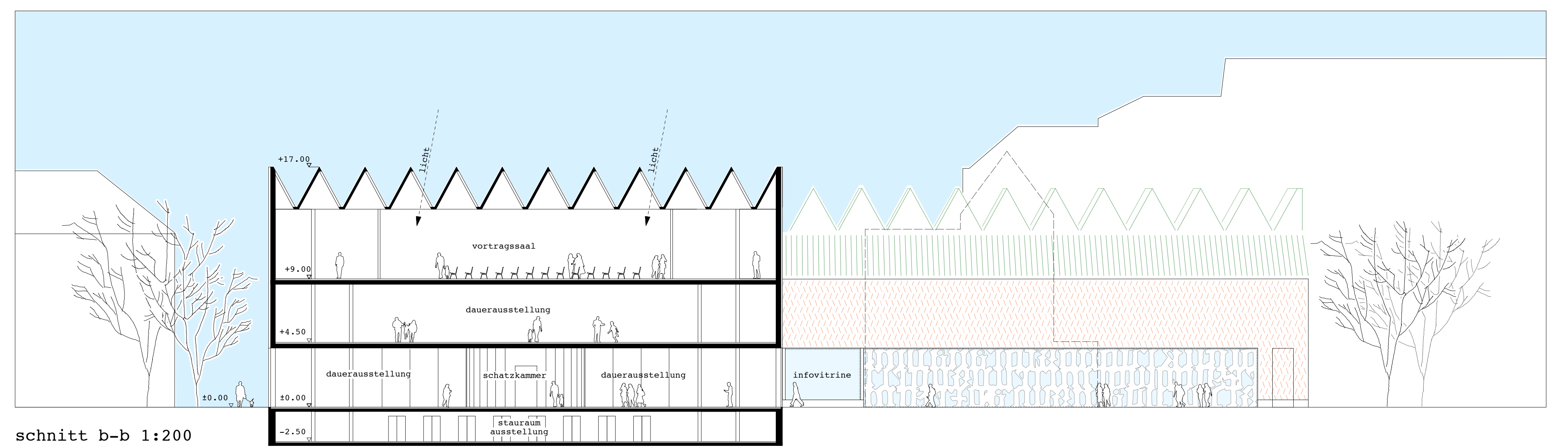
schnitt b-b 1:200
