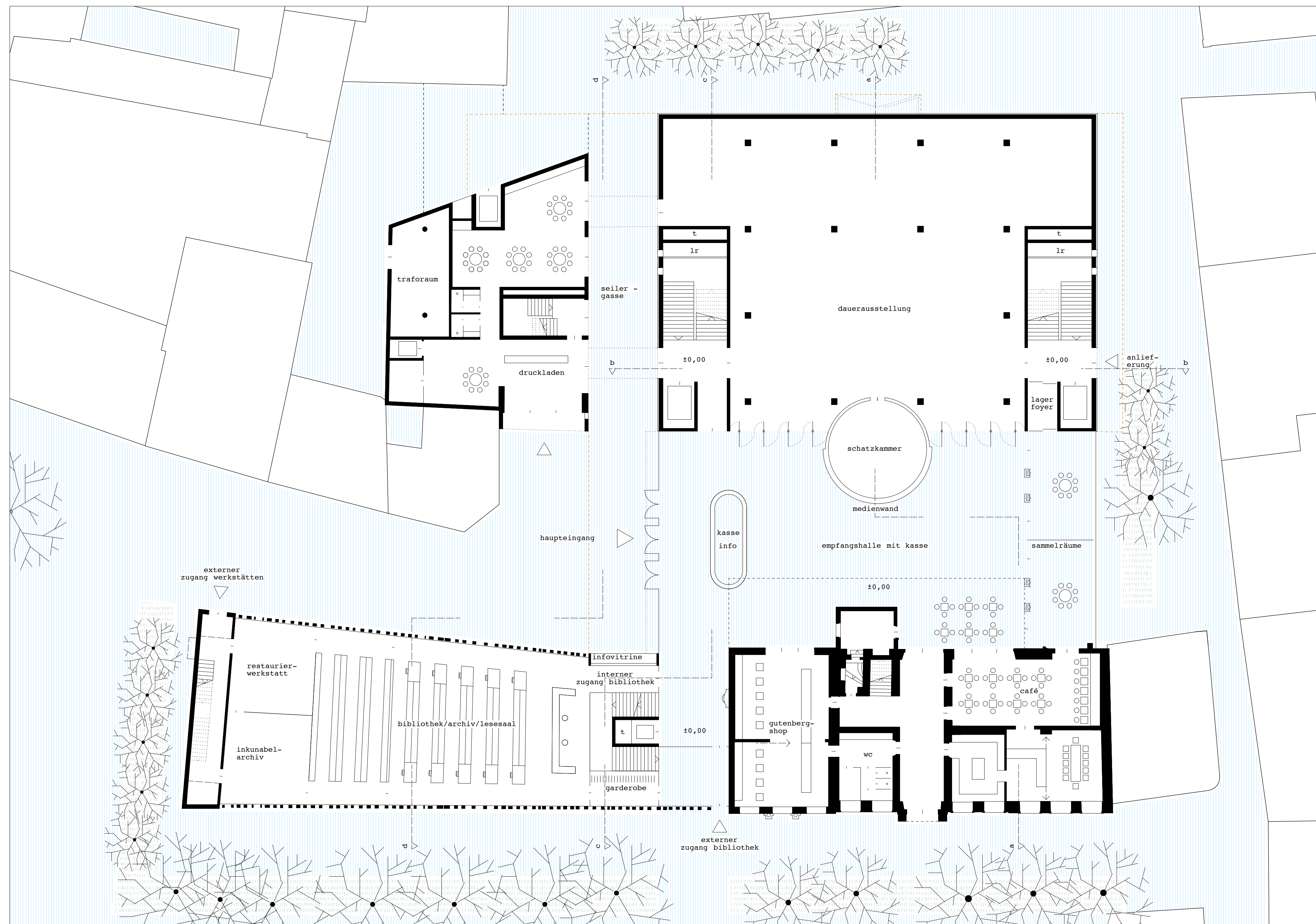
erdgeschoss 1:200
