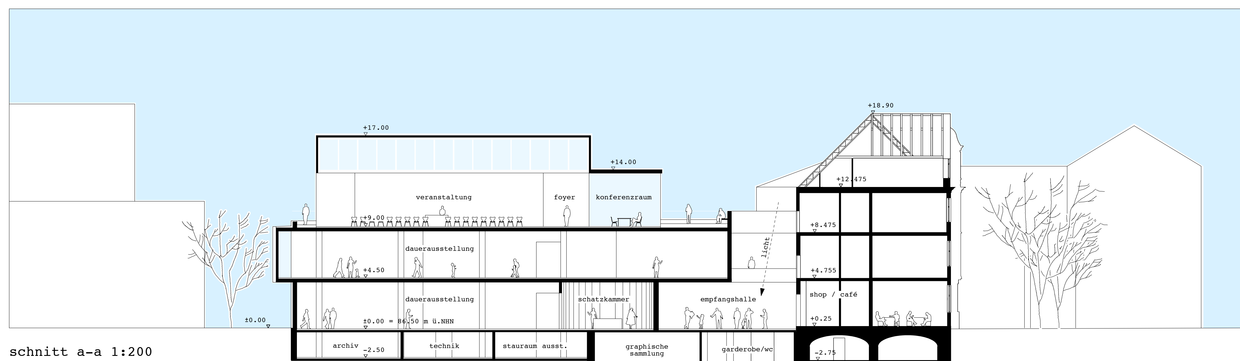
schnitt a-a 1:200
