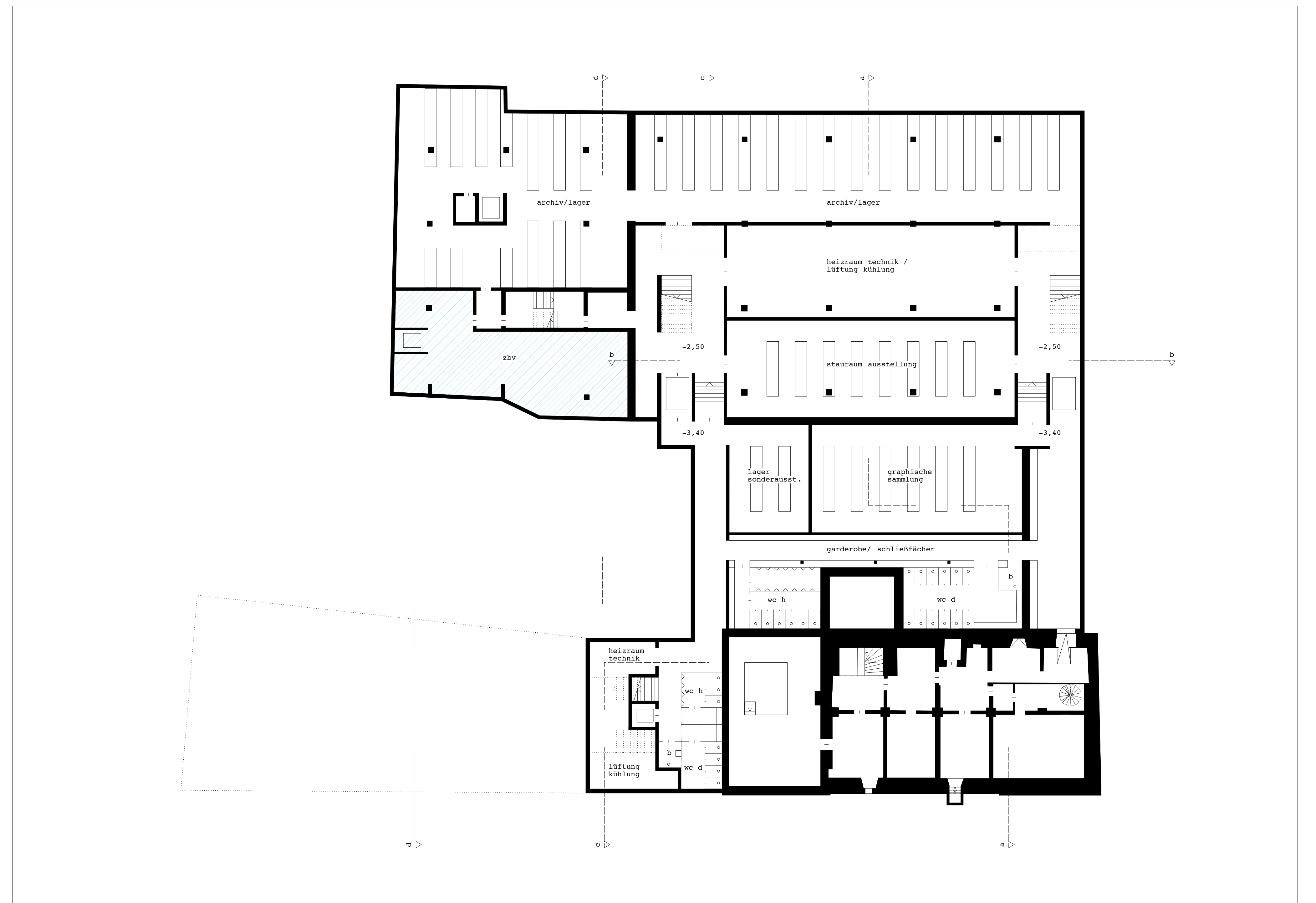
untergeschoss 1:200
